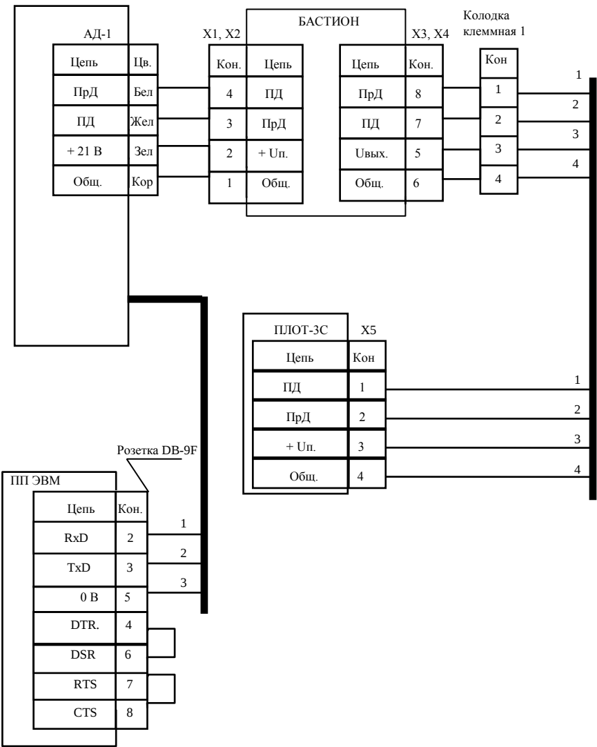
Схема электрическая соединений спиртомера с адаптером АД-1
