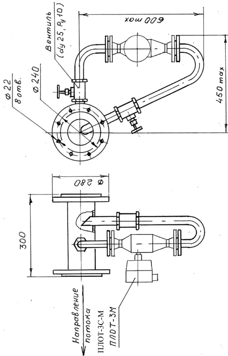
Пример установки спиртомера ПЛОТ-3С-М на горизонтальной трубе Ду 150
